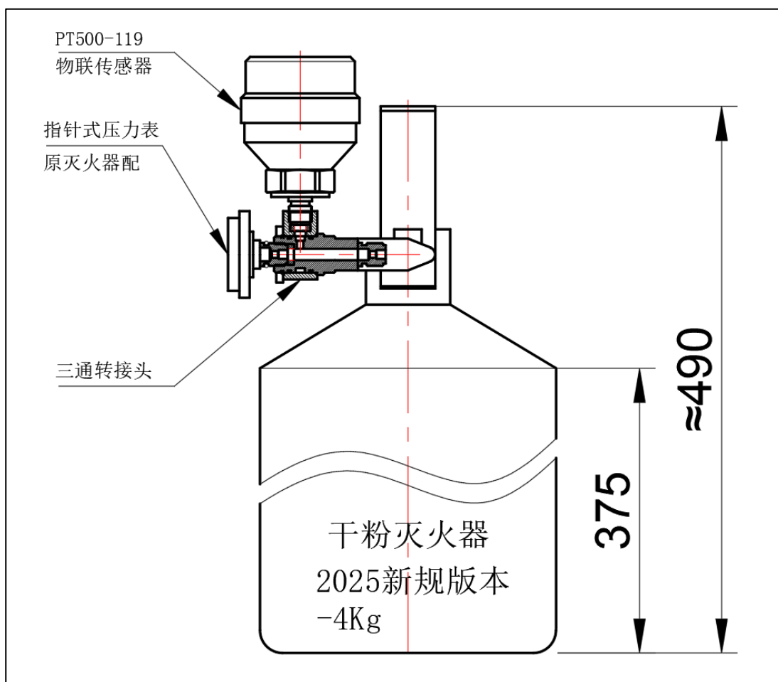
安装示意图
